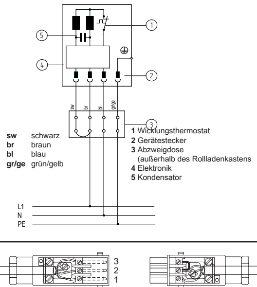
Fig. 5 Schaltbild SunTop/Z M-868 RH 230 V / 50 Hz und Kabelbelegung bei Verwendung mit Hirschmann-Steckverbindung STAS-3 (mit Brücke)
